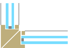
Illustration d'angle verre/paroi vitrée
