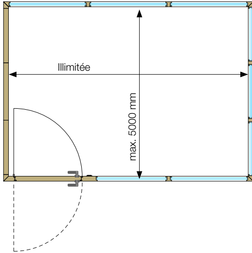
Illustration d'angle paroi pleine/monobloc
