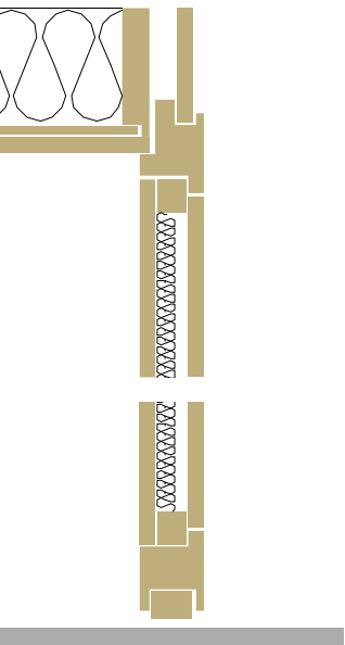
Paroi pleine double
