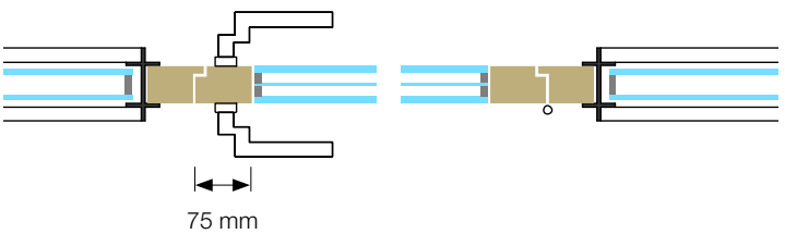
Porte en verre triple avec cadre bloc bois, montant 95 mm
