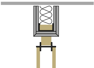
Retombée plâtre avec raccord au plafond
