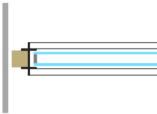
Raccord T avec lame sur cloison
