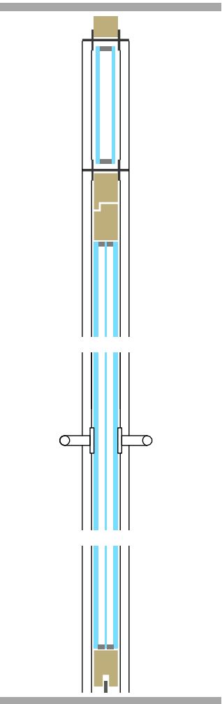
Porte en verre triple avec cadre bloc bois et imposte vitrée
