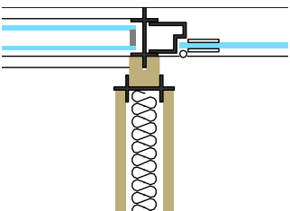
Angle droit modulable
