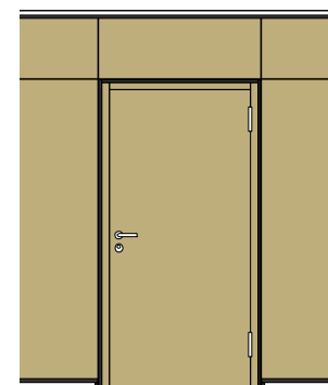
Cadre bloc bois avec imposte
