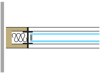
Raccord T avec porte
