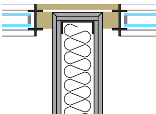
Raccord T sur mur avec habillage
