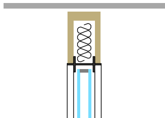
Raccord au plafond double
