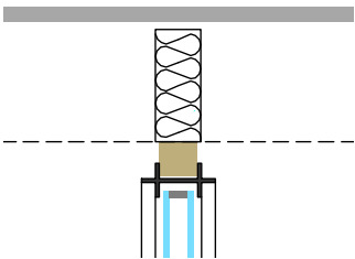
Isolation phonique faux-plafond
