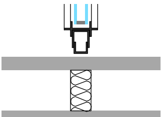
Isolation phonique sous plancher
