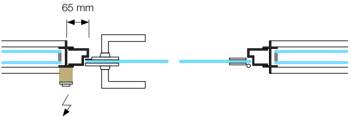
Porte en verre triple avec cadre bloc bois, montant 75 mm
