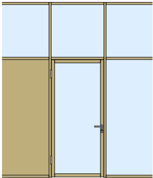
Montant de porte 99 mm, imposte vitrée EI0/EI30/EI60
