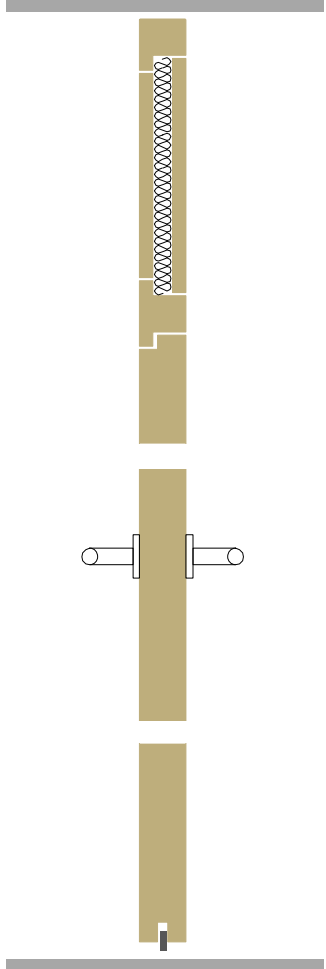
Porte pleine et imposte EI0/EI30
