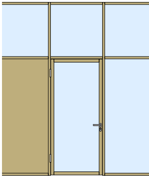
Montant de porte 81 mm, imposte vitrée EI0/EI30
