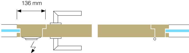
Porte pleine EI0/EI30
