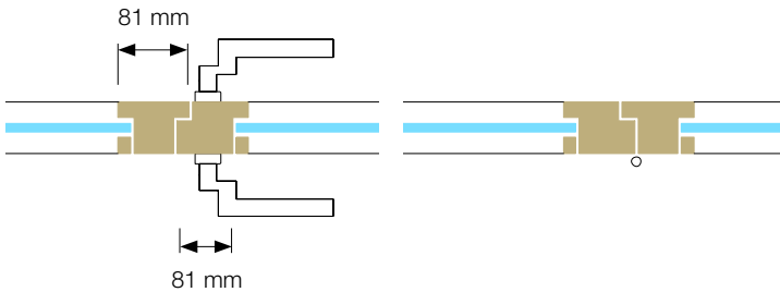
Porte bois-verre double, montant de porte 81 mm EI0
