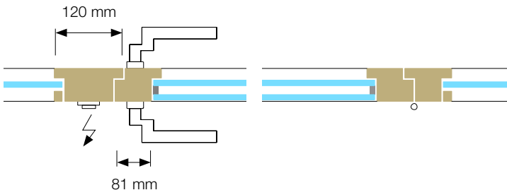
Porte pleine EI0/EI30
