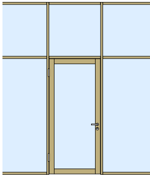
Montant de porte 120 mm, imposte vitrée EI0/EI30
