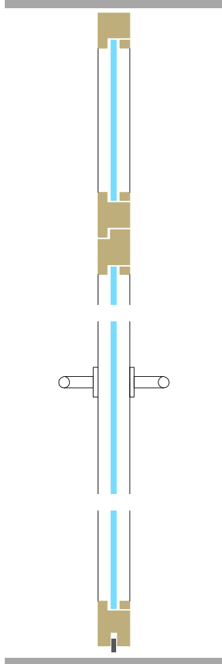
Porte bois-verre simple montant de porte 81 mm EI0/EI30
