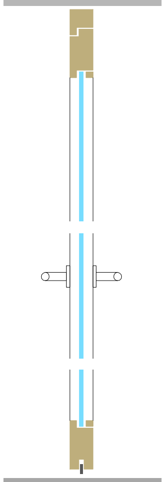
Porte bois-verre simple montant de porte 120 mm EI0/EI30
