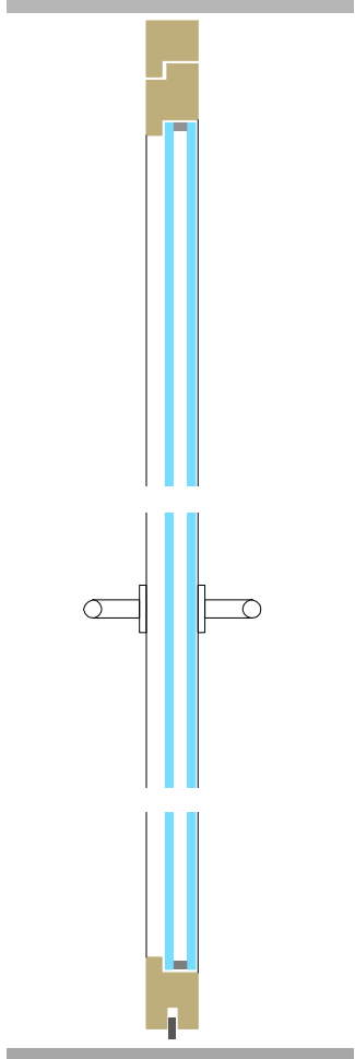
Porte bois-verre double montant de porte 81 mm EI0
