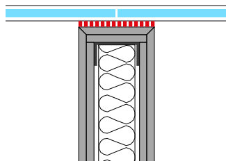
Raccord mural avec profilé
