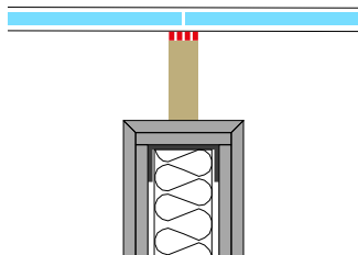
Raccord sur façade
