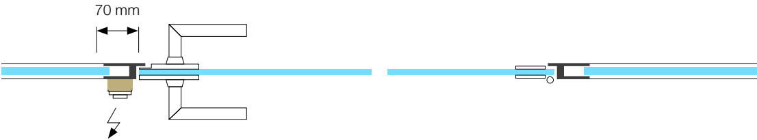
Porte en verre simple avec cadre aluminium
