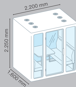
Meeting M (mit Sitztisch und Sitzbänke)
