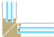
Eckausbildung Glas-/Glaswand
