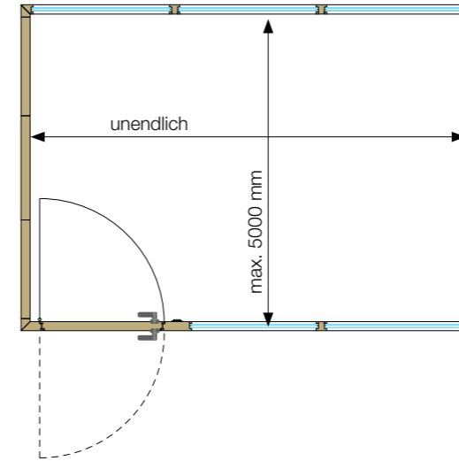
Eckausbildung Vollwand einschalig
