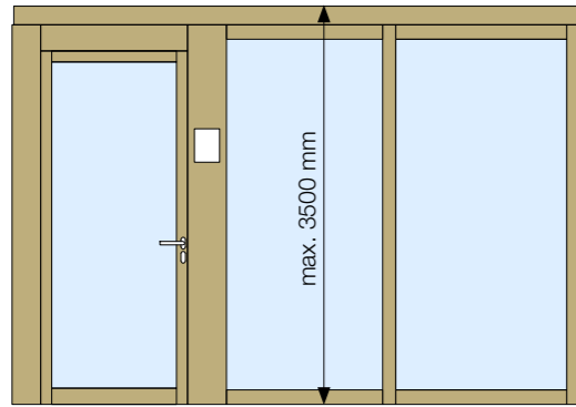
Ansicht aussen
