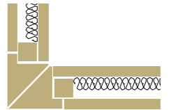
Eckausbildung Vollwand zweischalig
