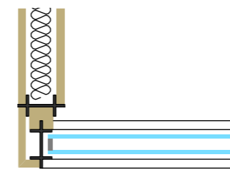
Eckausbildung 90° erweiterbar
