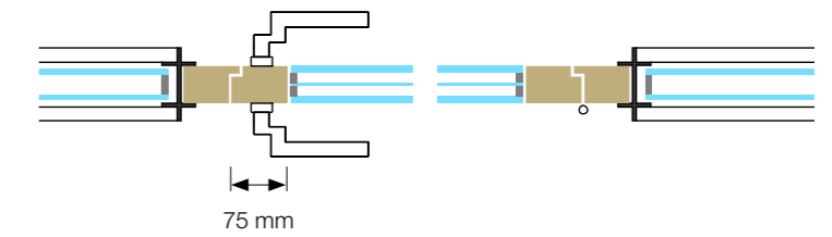
Isolierglastüre mit Holz-Blockrahmen, Flügelries 95 mm
