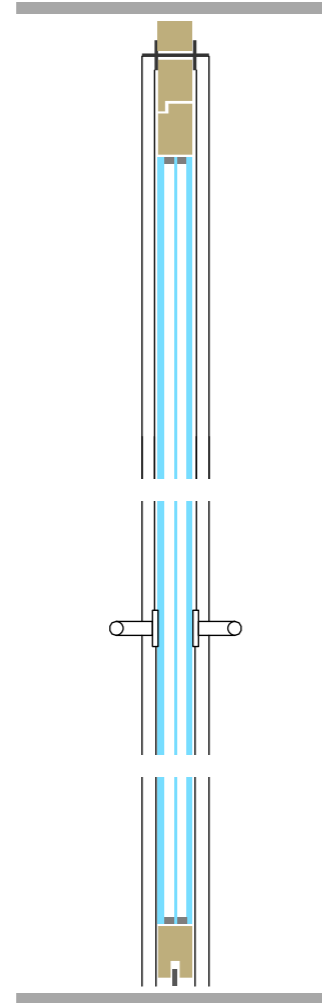
Isolierglastüre mit Holz-Blockrahmen
