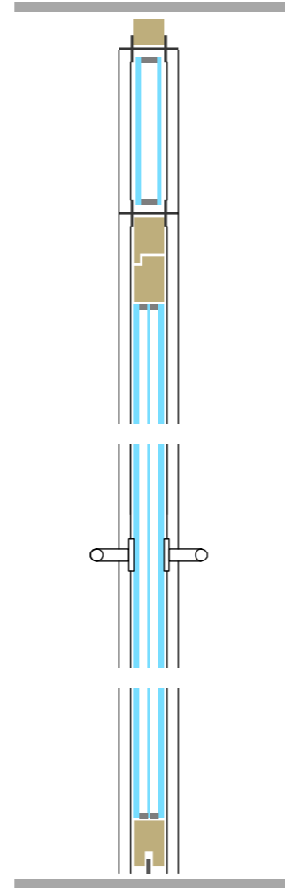
Isolierglastüre mit Holz- Blockrahmen und Glasoblicht
