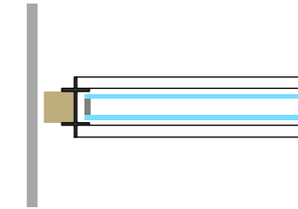
Querwandanschluss an Leichtbauwand
