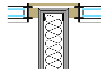
Querwandanschluss mit Stirnverkleidung
