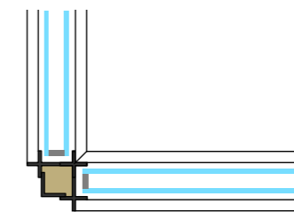
Eckausbildung 90°
