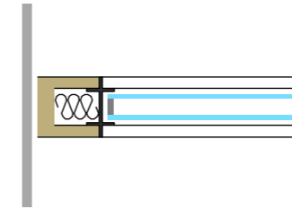
Wandanschluss zweischalig
