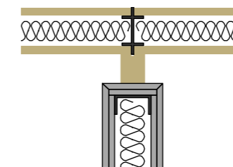
Querwandanschluss an Leichtbauwand
