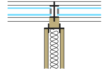
Querwandanschluss an Systemwand
