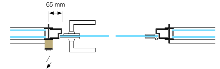
Isolierglastüre mit Holz-Blockrahmen, Flügelries 75 mm
