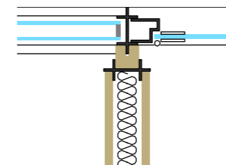
Querwandanschluss an Systemwand mit Tüorzarge
