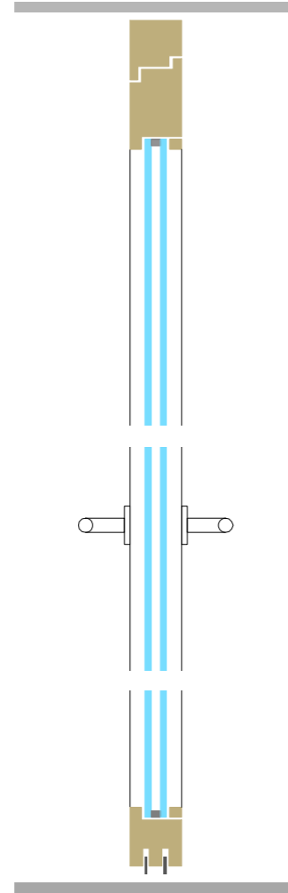
Holz-Isolierglastüre Flügelries 120 mm EI0/EI30
