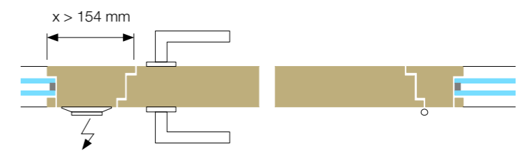
Volltüre EI0/EI30/EI60
