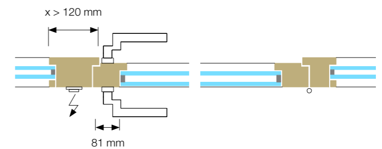
Volltüre EI0/EI30/EI60
