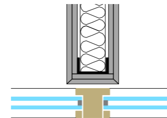
Querwandanschluss an Leichtbauwand EIO/EI60
