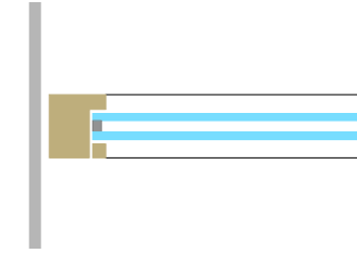
Eckausbildung 90° EIO/EI60
