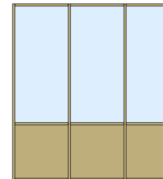
Brüstungswand, Pfosten-Riegel EI0/EI60
