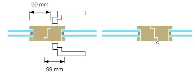
Holz-Isolierglastüre flächig, Flügelries 81 mm EI0
