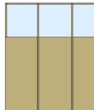
Oblichtwand, Pfosten EI0/EI60
