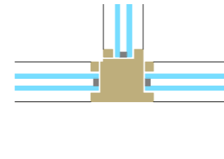
Querwandanschluss an Systemwand EIO
