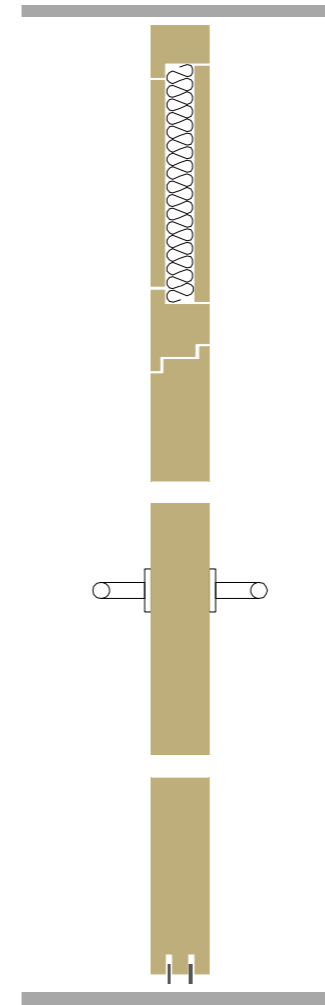
Volltüre EI0/EI30/EI60
