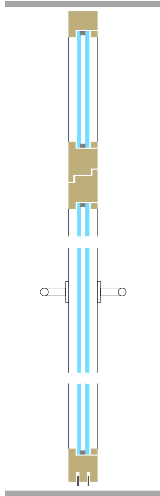
Holz-Isolierglastüre Flügelries 99 mm EI0/EI30
