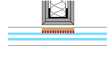
Eckausbildung variabler Winkel EIO
