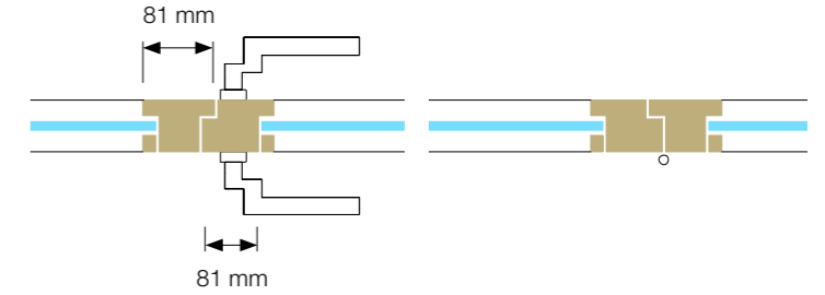
Holz-Isolierglastüre, Flügelstriebe 81 mm EI0
