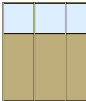
Oblichtwand, Pfosten-Riegel E10/EI30
