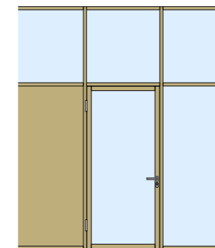
Flügelries 81 mm mit Glasoblicht EI0/EI30
