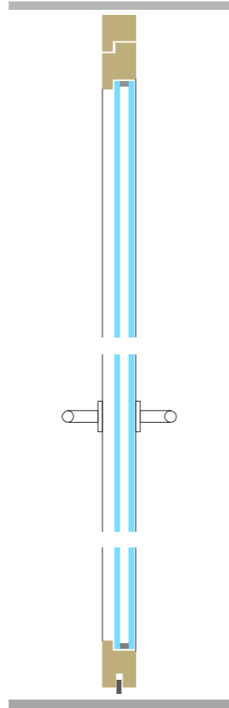
Holz-Isolierglastüre Flügelstriebe 81 mm EI0
