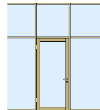
Flügelries 120 mm mit Glasoblicht EI0/EI30
