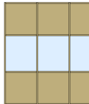
Mittelglaswand, Pfosten-Riegel E10/EI30
