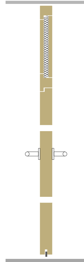
Volltüre mit Oberblende EI0/EI30
