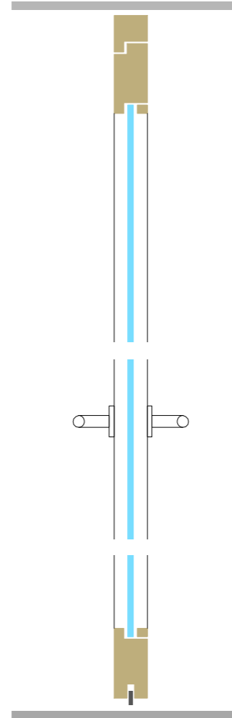
Holz-Glastüre VSG, Flügelstriebe 120 mm EI0/EI30
