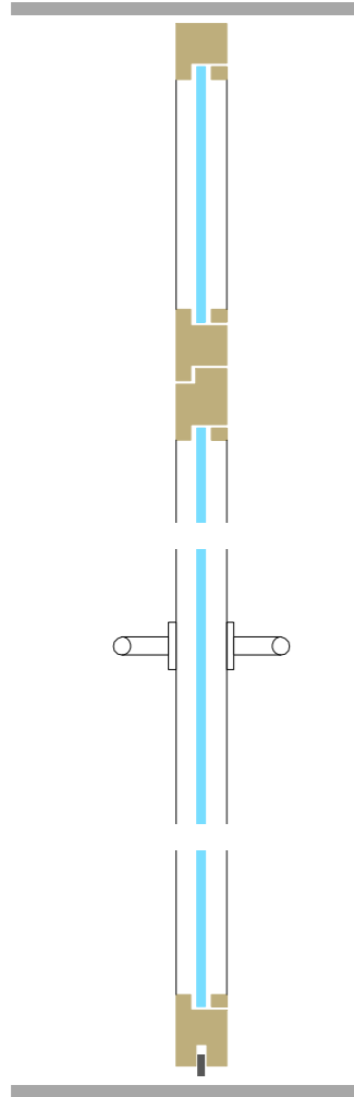
Holz-Glastüre VSG, Flügelstriebe 81 mm EI0/EI30
